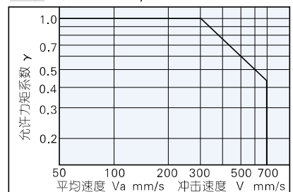
图线2 允许力矩系数: γ
