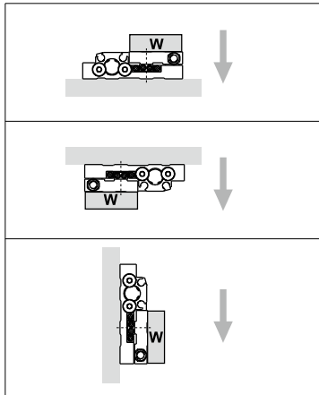
图1 集中负载质量: W(kg)
