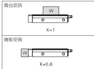
图3 工件安装系数: K
