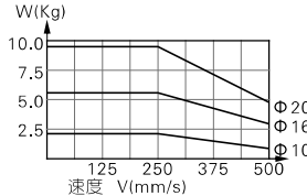
水平运行负载与速度关系曲线
