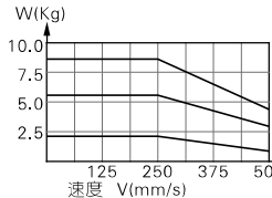
垂直运行负载与速度关系曲线
